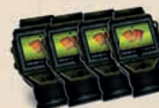
4 Geigerovy počítáče
